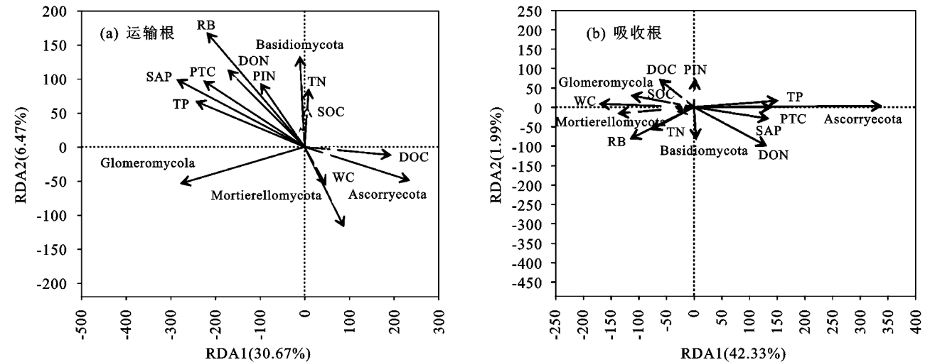
图 5 根系内生真菌影响因子 RDA 分析
