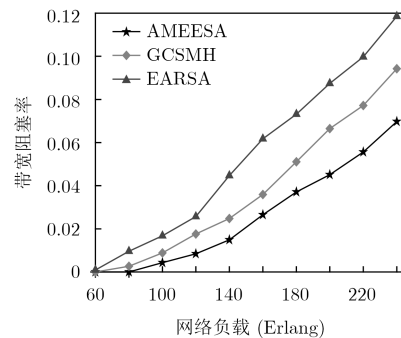
图4 不同负载条件下USNET网络中的带宽阻塞率
