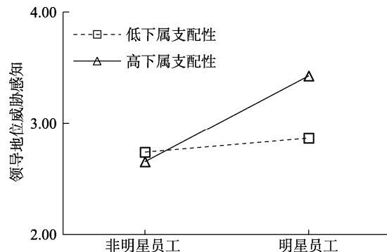
图 3 下属支配性对下属明星员工身份与地位威胁感知之间关系的调节作用
