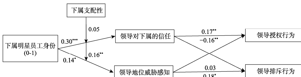
图4 研究2路径分析检验结果
