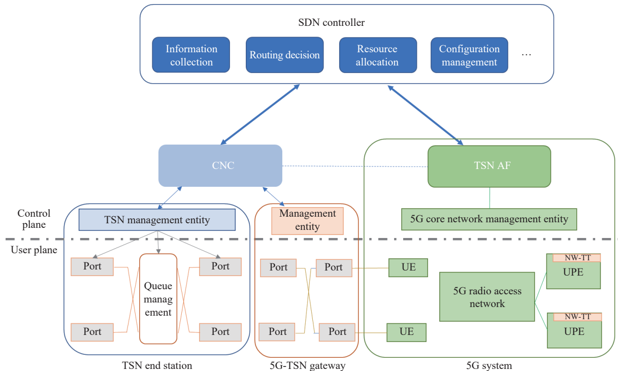
图 5 基于 SDN 的 5G-TSN 管控架构 Fig.5 SDN-based 5G-TSN management architecture
