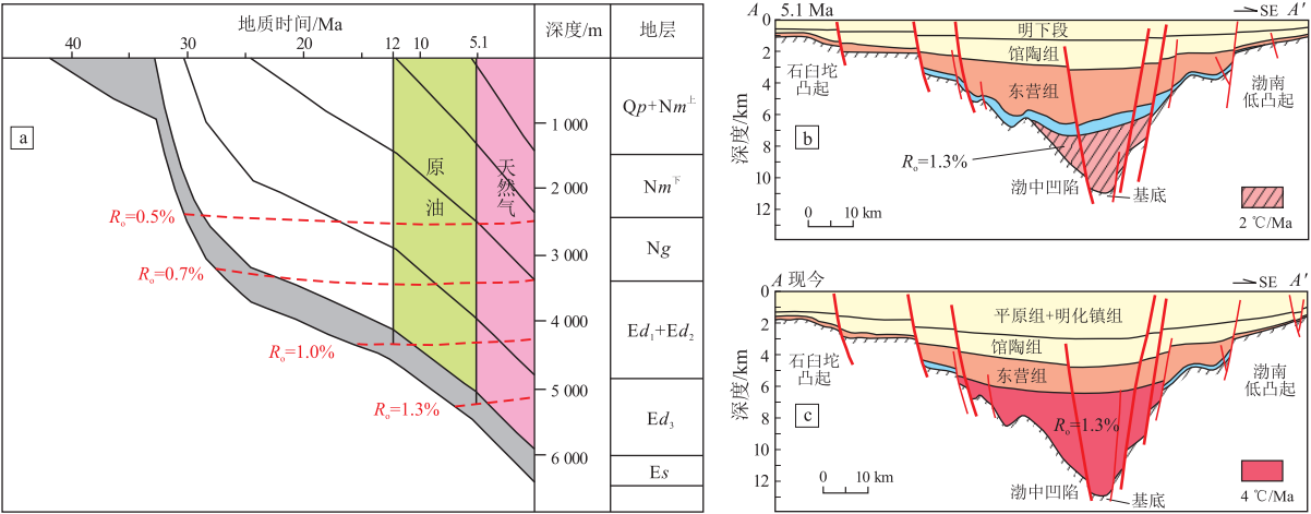
图 5 渤海湾盆地渤中烃源岩热演化史(a)与 5.1 Ma 前后生气面积变化(b,c)
