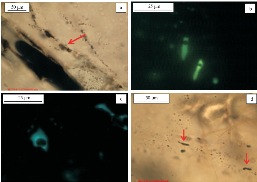
图6 渤海湾盆地渤中凹陷 BZ19-6 凝析气藏原油及气包裹体镜下显微特征 a.BZ19-6-1 井,3 735 m,褐色重质油包裹体,单偏光;b.BZ19-6-1 井,3 735 m,黄绿色轻质油包裹体,荧光; c.BZ19-6-1 井,3 735 m,蓝白色轻质油包裹体,荧光;d.BZ19-6-1 井,4 106 m,灰色天然气包裹体,单偏光
