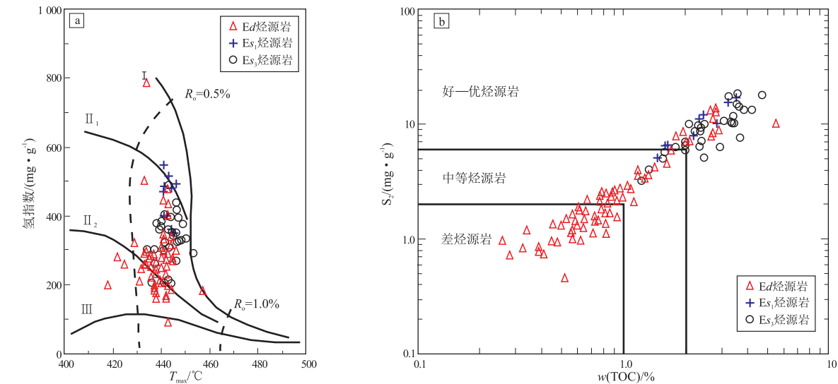
图2 渤海湾盆地渤中凹陷 BZ19-6 构造烃源岩有机地球化学特征
