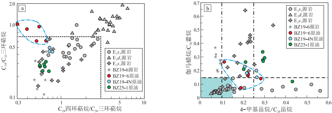
图 4 渤海湾盆地渤中凹陷 BZ19-6 凝析气藏原油的生源参数组成及油源划分
