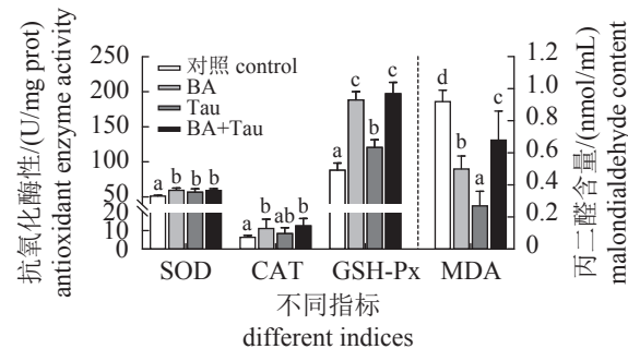
图 1 胆汁酸和牛磺酸对大口黑鲈肝脏抗氧化指标的影响
