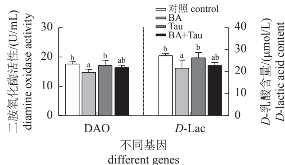
图 8 胆汁酸和牛磺酸对大口黑鲈肠道通透性的影响
