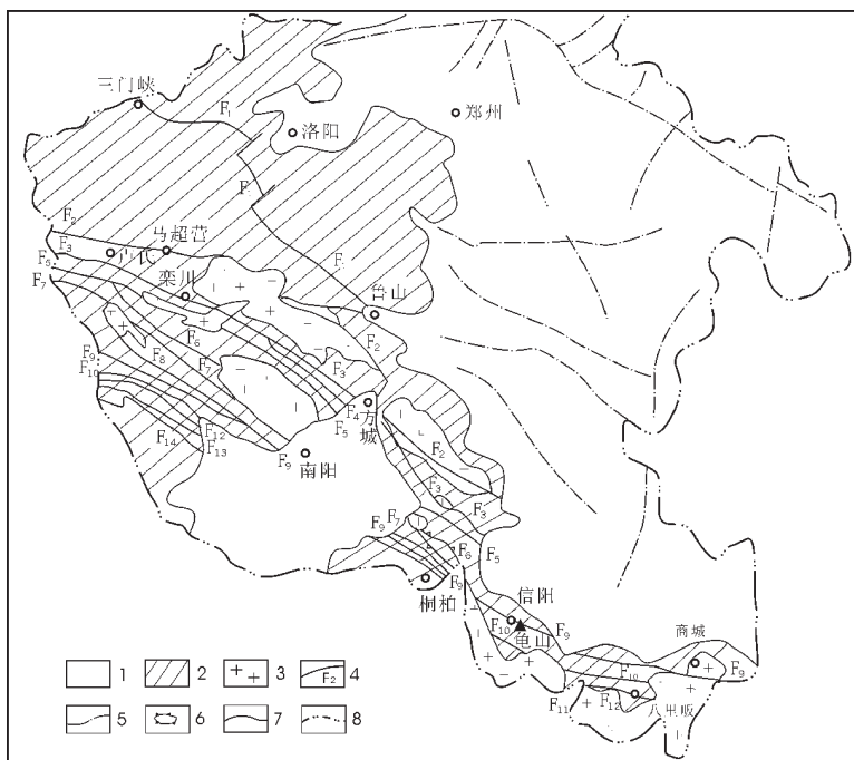
图1 河南省主要构造分布图(据王志宏,2000修编)
