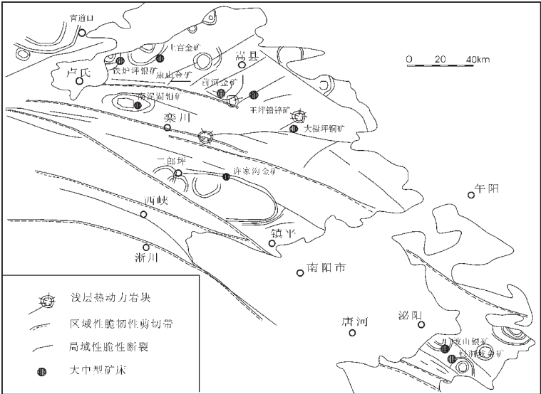
图 3 卢氏—桐柏地区遥感解译图
