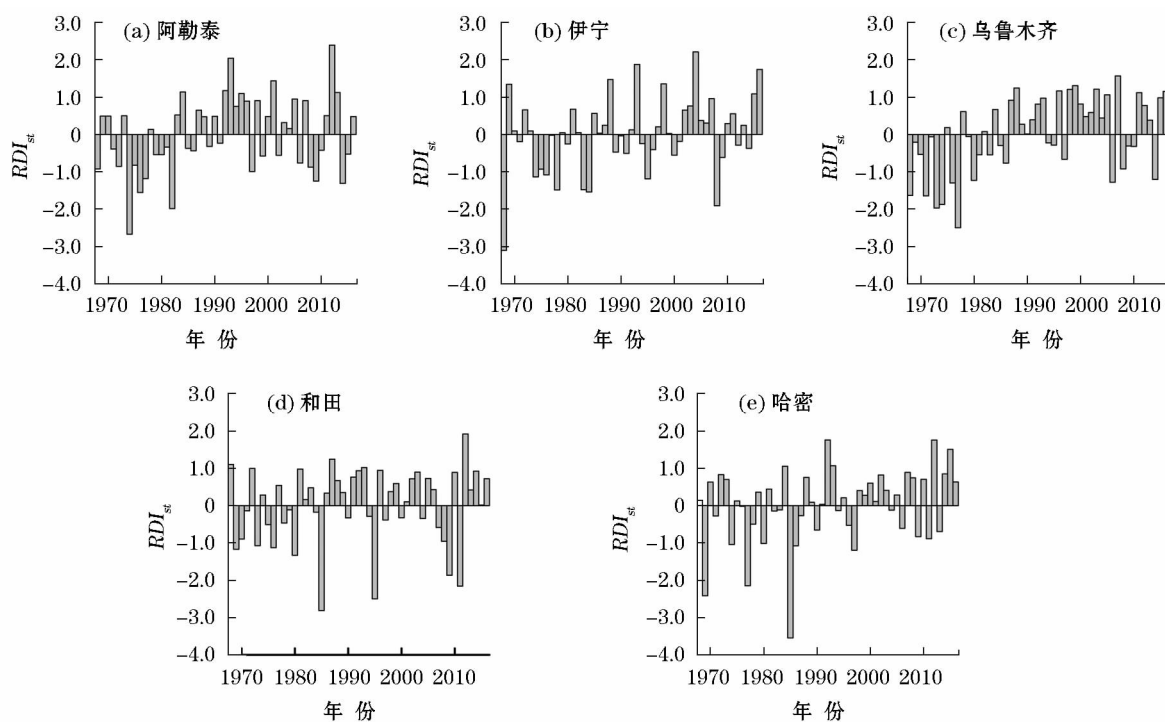
图 5 新疆 5 个代表站年尺度 RDI_{st} 变化特征
