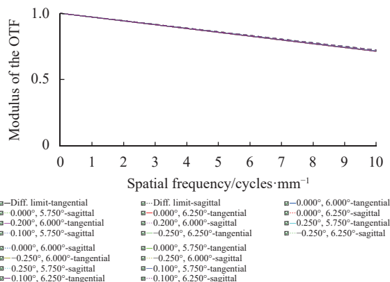
图 6 某测试用平行光管的 MTF 曲线
