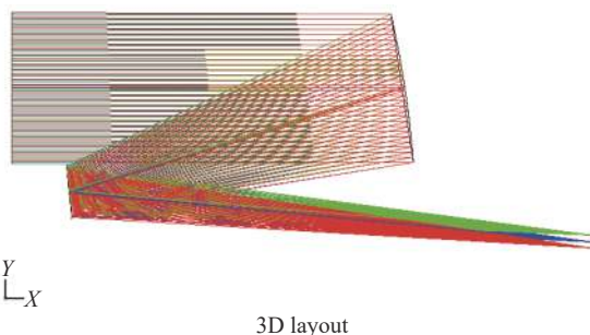
图 5 某测试用平行光管光路图
