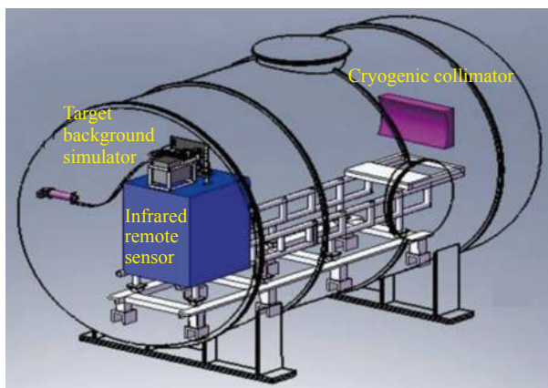
图 4 探测信噪比测试设备布局位置图
