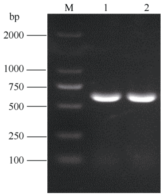
图 1 PCR 电泳结果。M: DNA marker 2000; 1, 2: ArCRC 基因全长 CDS。
