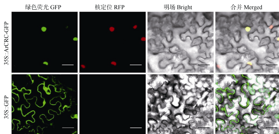
图 4 ArCRC 蛋白在烟草叶片下表皮细胞中的亚细胞定位。标尺=25 \mu m
