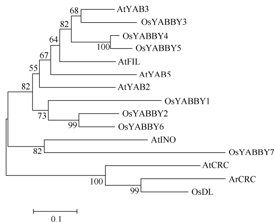
图 3 ArCRC 与水稻和拟南芥 YABBY 蛋白聚类分析
