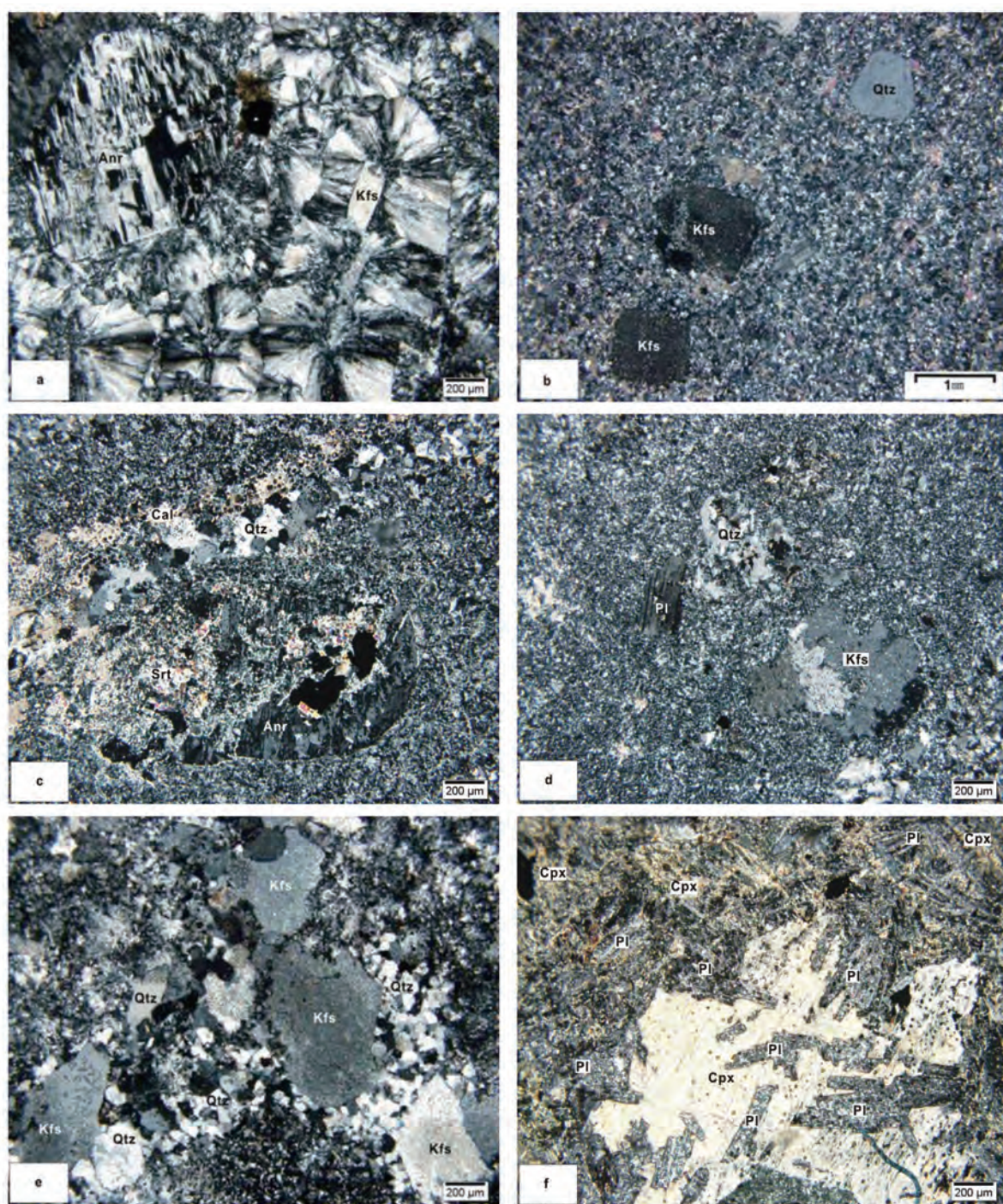
图3 鸡冠山钼矿区岩石样品显微照片
