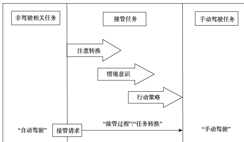
图1 接管过程(资料来源: Ito et al., 2016)
