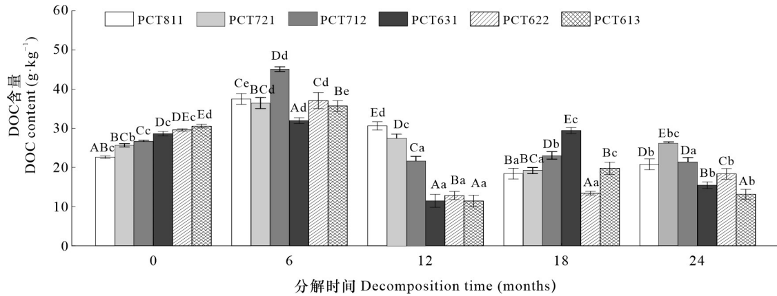
图3 一针两阔凋落叶的 DOC 含量的动态变化
