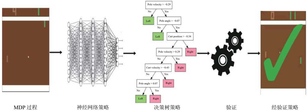
图5 决策树等价模型验证方法流程
