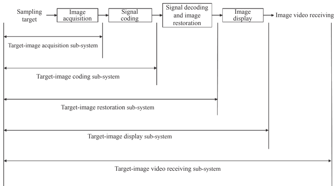
图 6 采样成像系统的若干子系统划分
