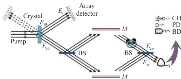
图 14 全息鬼成像原理示意图 [93]
