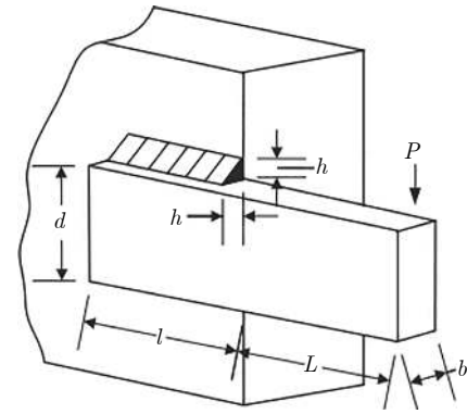
图 9 焊接梁模型
