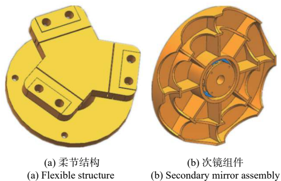
图 8 柔节结构及次镜组件
