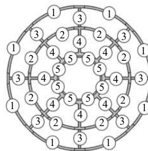
图 6 轻量化筋分组示意图
