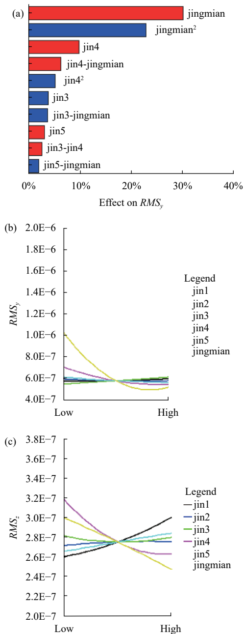
图 7 Paroto 图和主效应图
