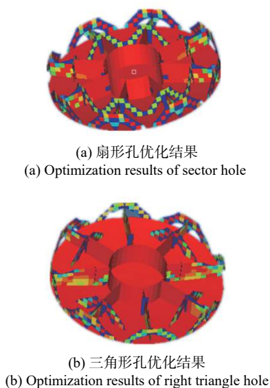
图 4 基结构拓扑优化结果
