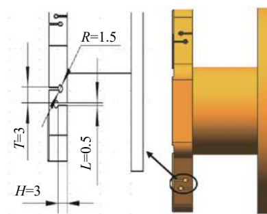
图 9 柔节优化参数
