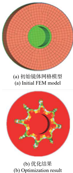
图 2 实体镜模型及优化结果 Fig.2 Solid mirror model and optimization result
