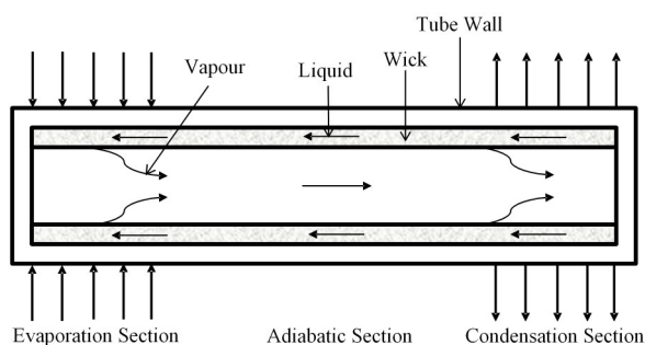
图8 热管工作原理示意
