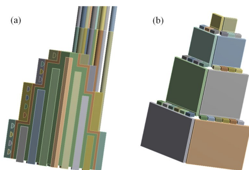
图7 简化后的1/3模型(a)和发电片结构(b)
