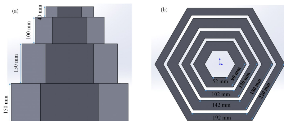
图6 冷端座示意及参数 (a) 正视图, (b) 俯视图
