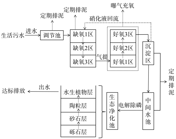
图 1 工艺流程
