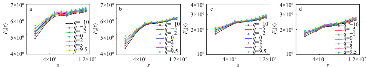
图 4 南海 SST 序列的时间尺度 s 与波动函数 F_q(s) 的双对数
