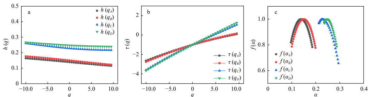
图5 南海不同海域 SST 序列 MFDFA 分析结果
