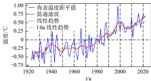
图1 南海百年海表温度变化趋势
