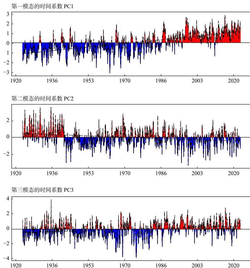
图2 南海 SST EOF 分析时间系数变化图
