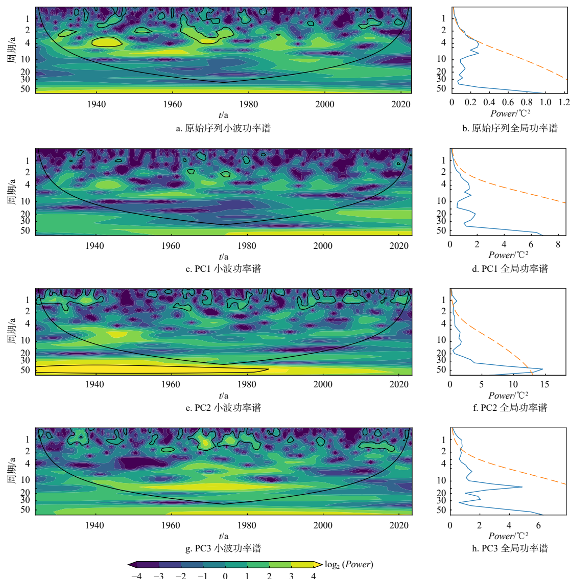
图 3 南海 SST 原始序列及 EOF 分解三种时间系数小波分解图
