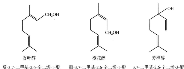
图 3 香料单体结构图
