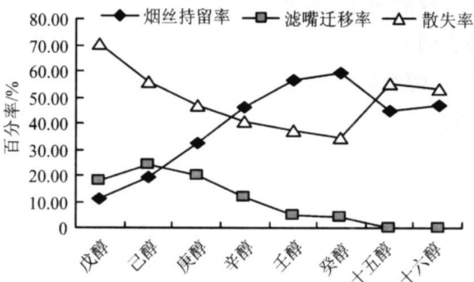
图 1 醇类同系物香料加香抽吸前的转移情况
