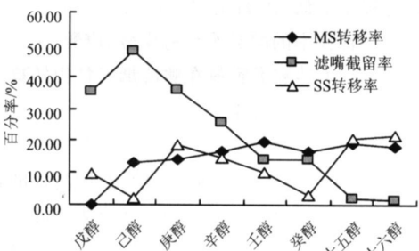
图 2 醇类同系物香料加香抽吸后的转移情况
