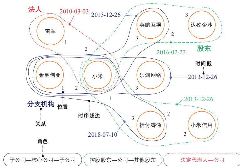
图 1 时序知识超图示例
