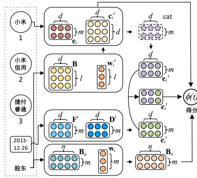
图 2 THM 总体架构图
