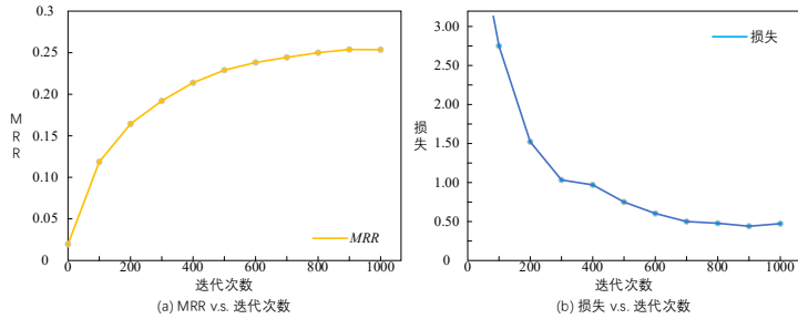
图 4 从 MRR 和损失指标分析过拟合现象
