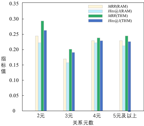
图 3 不同关系元数下的细分性能
