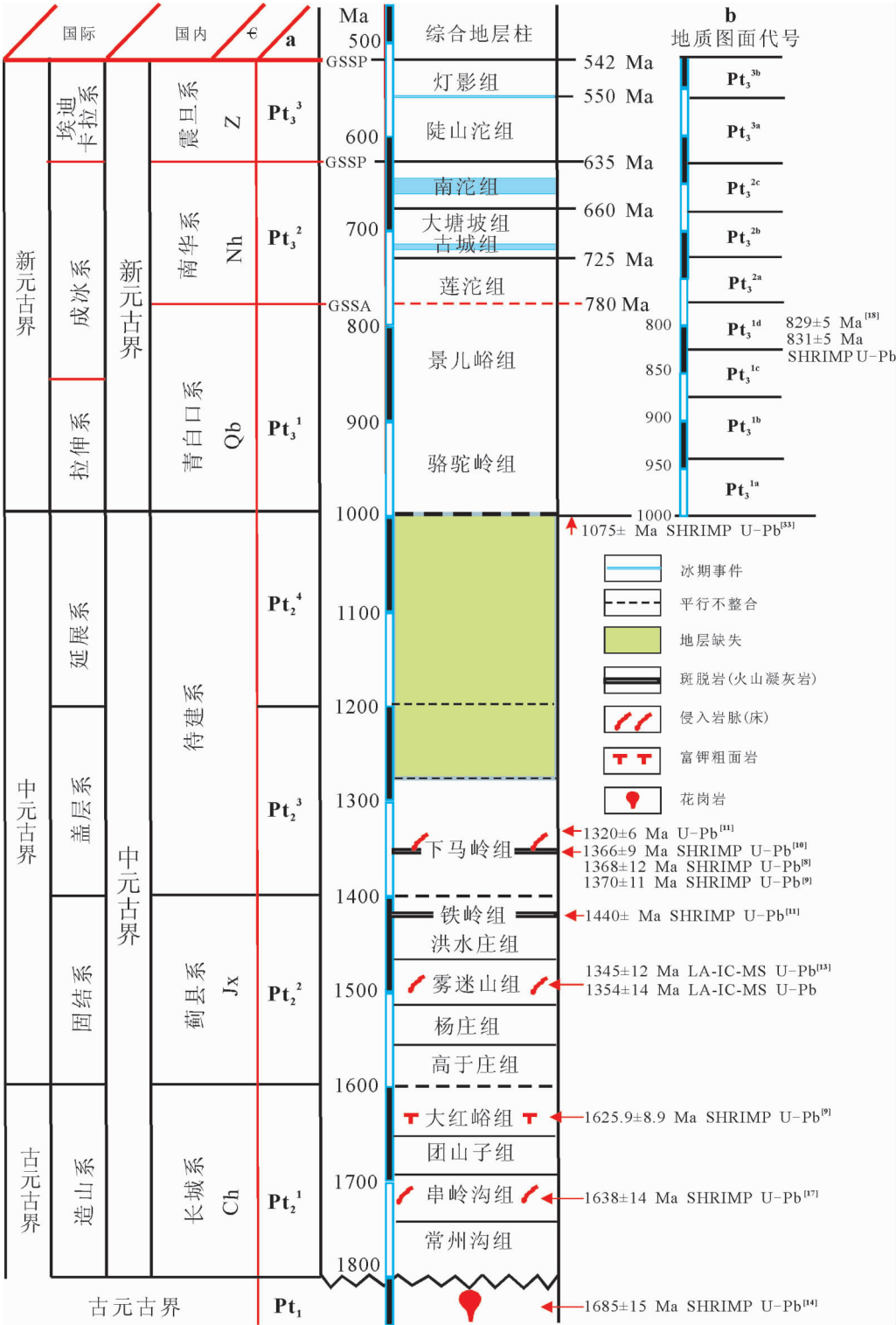
图 1 中国晚前寒武系综合柱状图 Fig.1 Late Precambrian stratigraphic column of China
