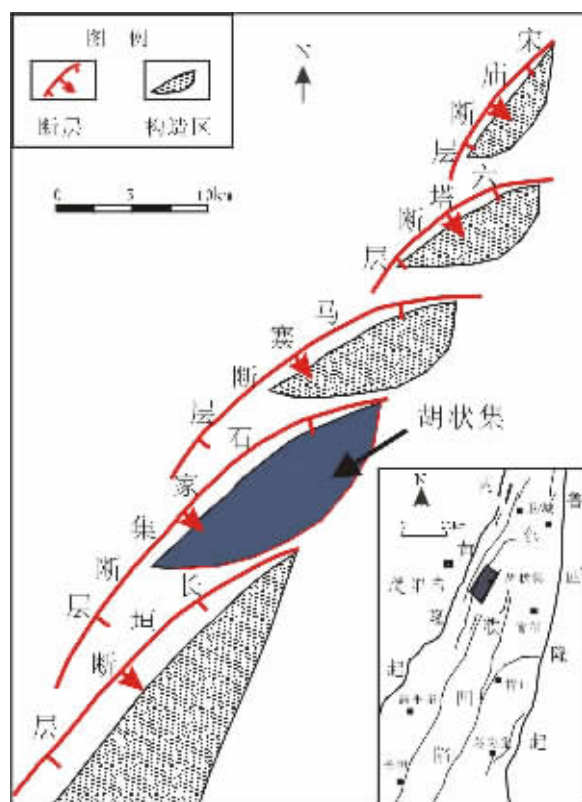
图 1 河南濮阳胡状集油田构造位置略图
