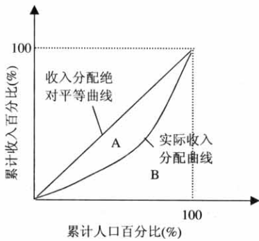
图 1 洛伦茨曲线
