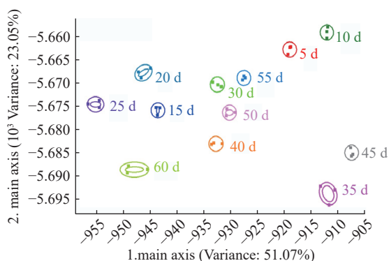
图9 粗鱼油挥发性气味在37℃贮藏条件下的LDA图
