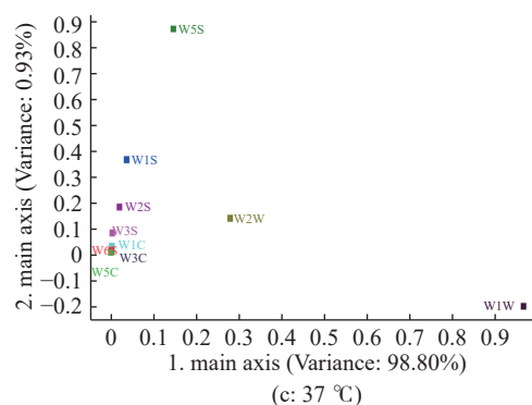
图10 粗鱼油挥发性气味在不同贮藏温度条件下的载荷分析图
