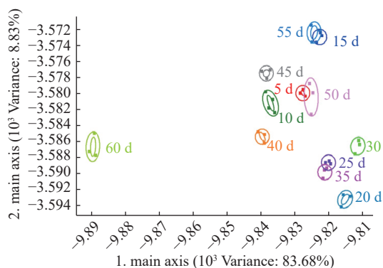
图7 粗鱼油挥发性气味在4℃贮藏条件下的LDA图
