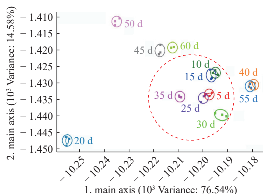
图8 粗鱼油挥发性气味在25℃贮藏条件下的LDA图
