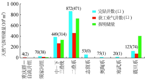
图 1 蜀南地区各层系勘探成效简图
