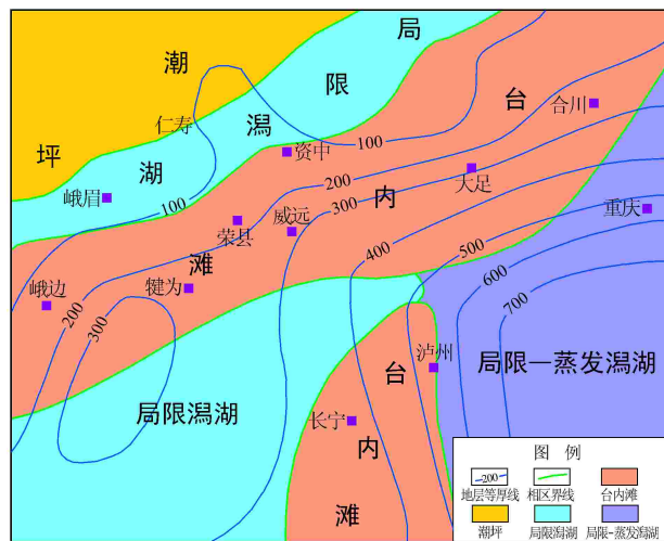
图2 蜀南地区早寒武世龙王庙期岩相古地理图
