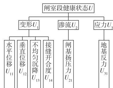
图 2 东溪水闸闸室段健康诊断指标体系 Fig. 2 Health diagnosis index system for Dongxi sluice chamber section
