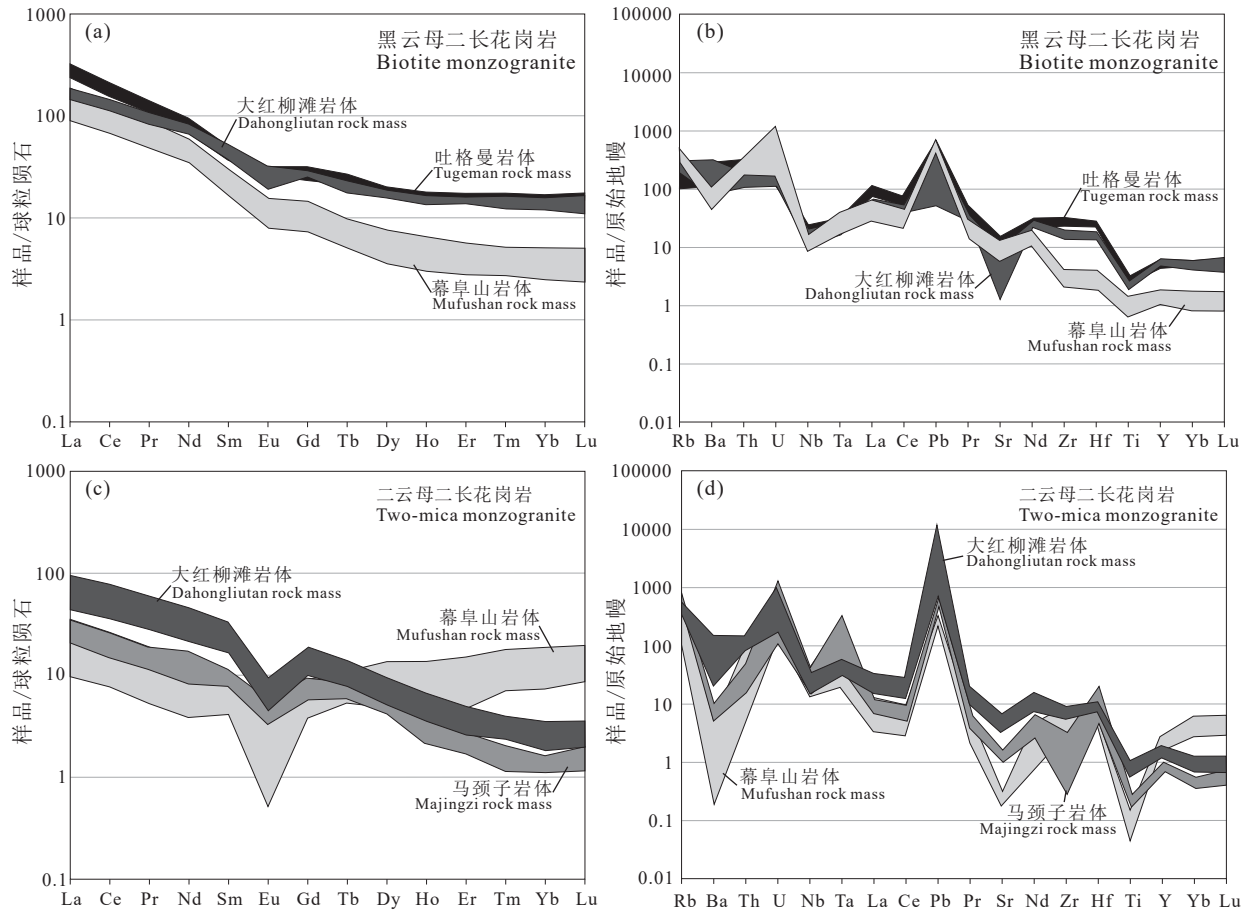
图5 中国主要花岗伟晶岩型锂矿(田)产锂花岗岩石球粒陨石标准化稀土元素配分图(a, c)和原始地幔标准化微量元素蛛网图(b, d)
