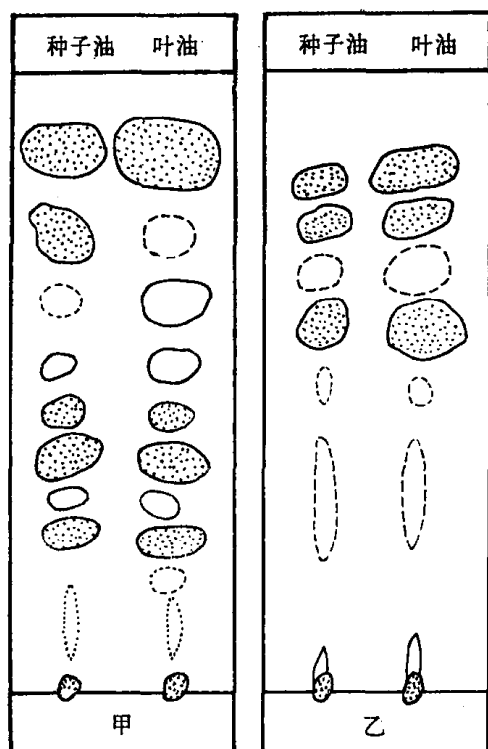
图1 两种砂仁挥发油薄层层离谱
