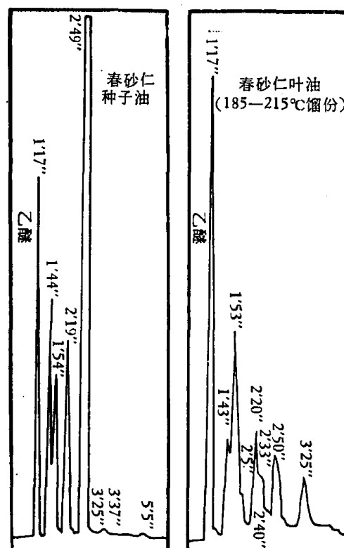
图2 两种砂仁挥发油气相色谱
