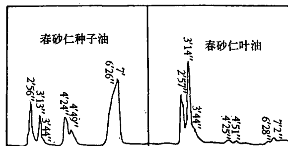
图3 两种砂仁挥发油气相色谱
