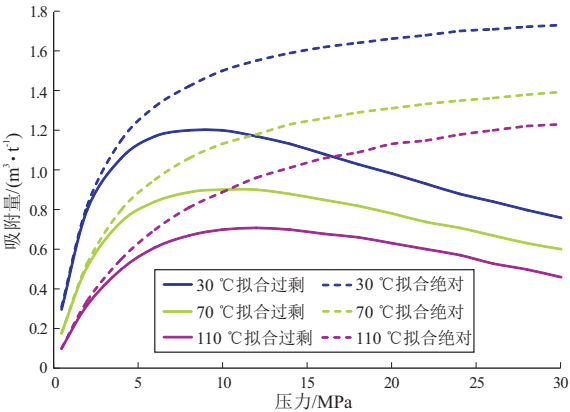
图3 川东南 JY7 井龙马溪组深层页岩样品在不同温度下的拟合过剩吸附量与绝对吸附量
