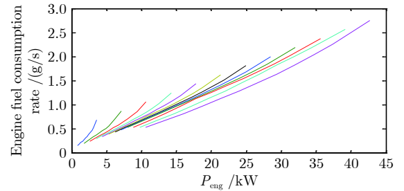
图 4 发动机燃油消耗率-功率曲线
