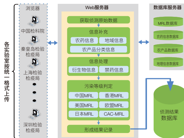
图 4 农药残留侦测数据采集系统架构图
