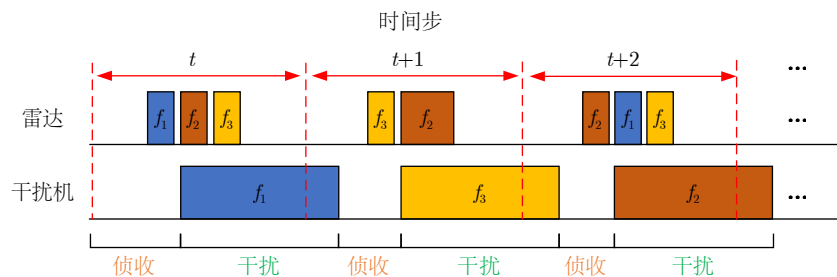
图5 脉内侦干策略
