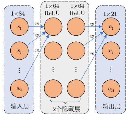
图4 全连接神经网络结构示意图
