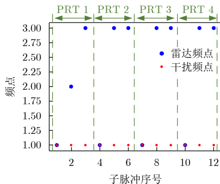
(a) 雷达子脉冲频点和干扰频点选取
