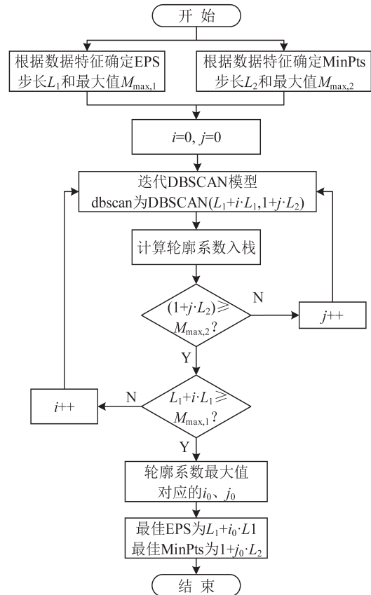
图 4 A-DBSCAN 聚类算法流程
