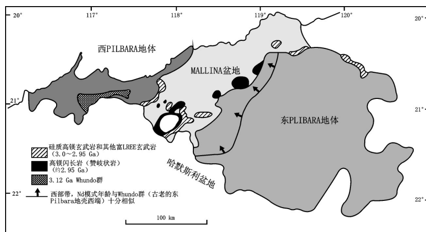
图3 西Pilbara地体和Malina盆地中富镁岩浆单元俯冲带
