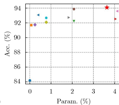
(b) Swin-Tiny模型上RESISC45数据集的对比试验结果
