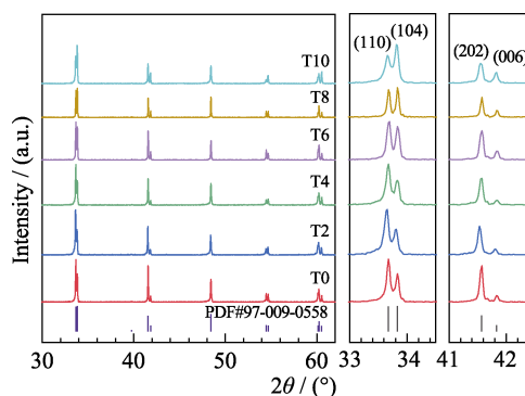
图 2 不同 TEOS 浓度的 \text{PrAlO}_3 陶瓷 XRD 谱图
