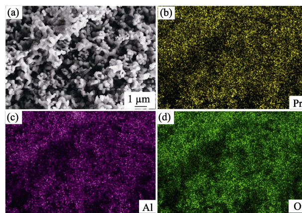
图 4 1200\text{ }^\circ\text{C} , \text{Ar}/\text{H}_2 气氛下烧结的 \text{PrAlO}_3 的 SEM-EDS 照片和各元素分布图
