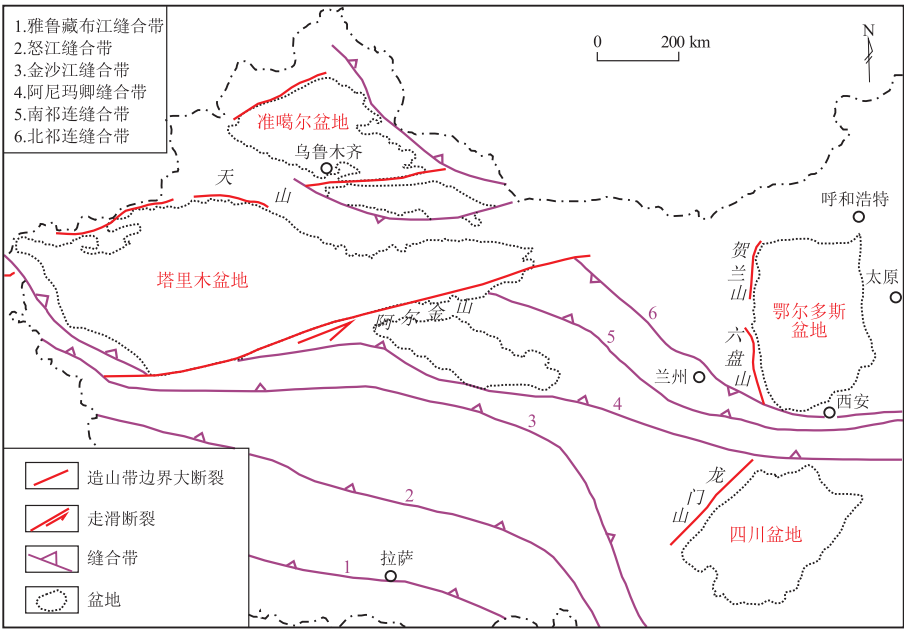
图 1 中国中西部主要盆地分布
