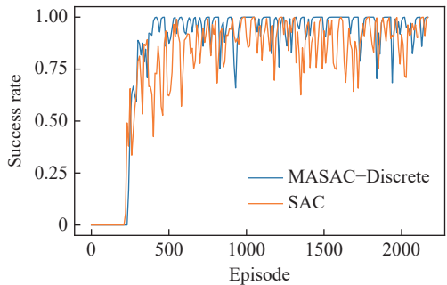
图 4 任务成功率曲线 Fig.4 Task success rate curve
