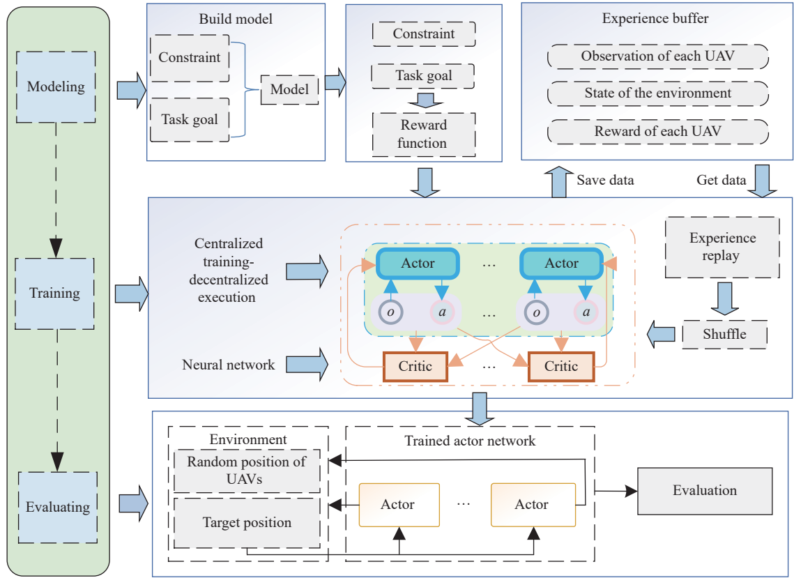
图 1 多无人机协同探索方法实施框架
