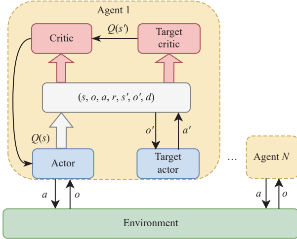
图2 MASAC-Discrete 算法架构
