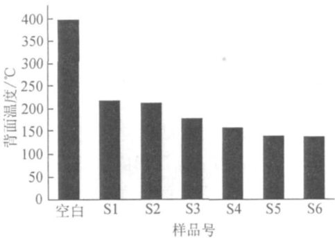
图 2 不同样品的钢板背面温度 Fig.2 Back temperatures of different samples
