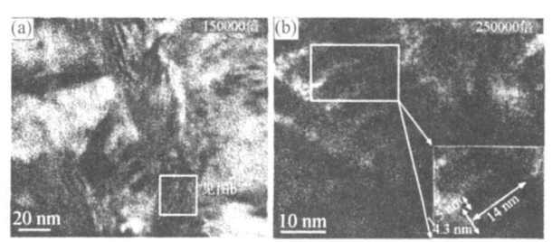
图 8 氨基树脂/OMMT 纳米插层复合物的 TEM 图 Fig.8 TEM images of amine resin/OMMT nanocomposite
