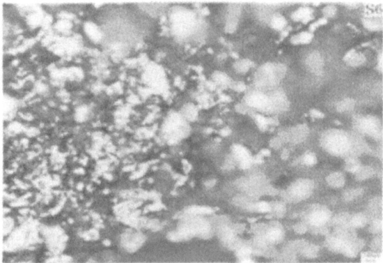
图 1 膨胀炭层显微图 Fig.1 SEM image of intumescent char
