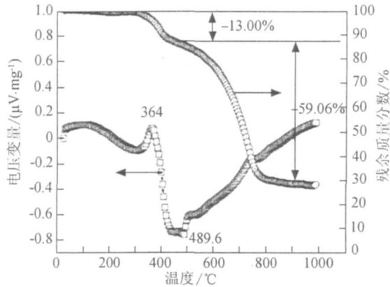
图 3 脱水成炭催化剂的 TG, DTA 曲线 Fig.3 TG and DTA curves of dehydration peat-forming catalysts
