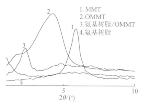
图 7 MMT 及氨基树脂/OMMT 纳米插层复合物的 XRD 图 Fig.7 XRD curves of MMT and amine resin/OMMT nanocomposite
