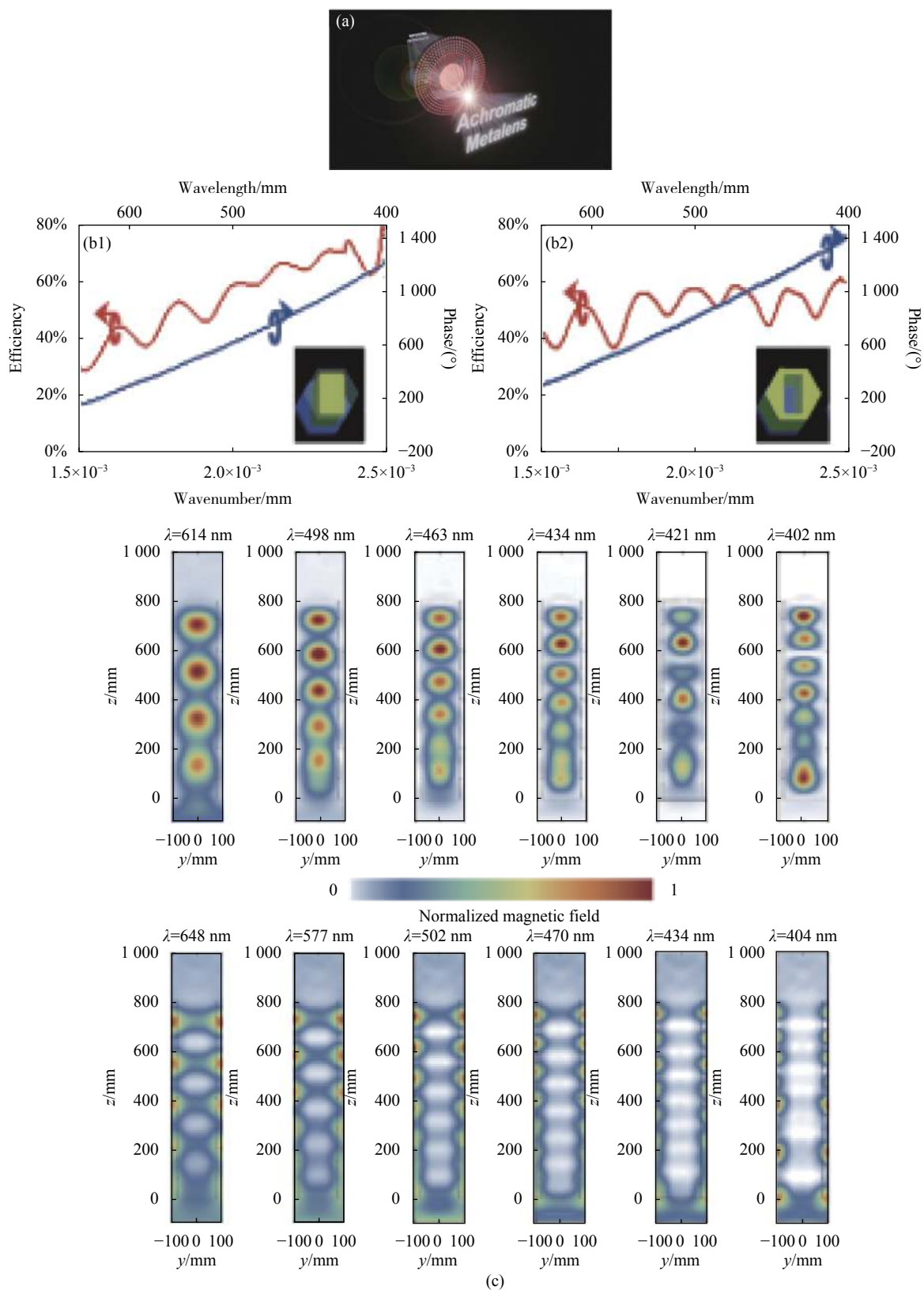
图 3 (a) 可见光宽带消色差超构透镜示意图; (b) 介质柱结构和介质槽结构对应的相位曲线 (蓝色曲线) 和工作效率 (红色曲线); (c) 超透镜单元中不同入射波长的归一化磁能 [40]
