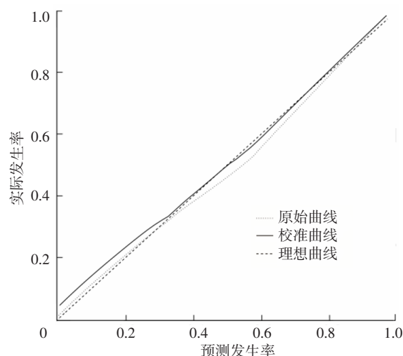
图2 列线图模型预测建模集癫痫患者发生睡眠障碍的校准曲线
