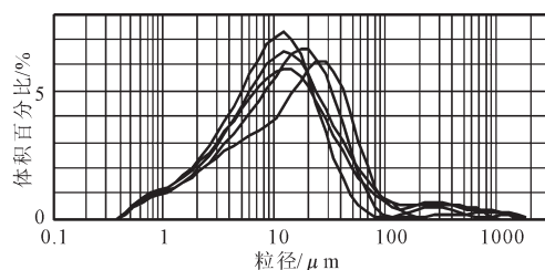
图2 2006年3月哈尔滨5个沙尘沉降物的粒度分布曲线 Fig.2 Grain-size distribution of sand-dust fallouts in Harbin in March 2006
