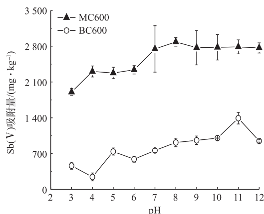
图3 不同pH对Sb(V)吸附影响
