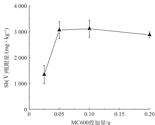
图2 MC600投加量对Sb(V)吸附影响
