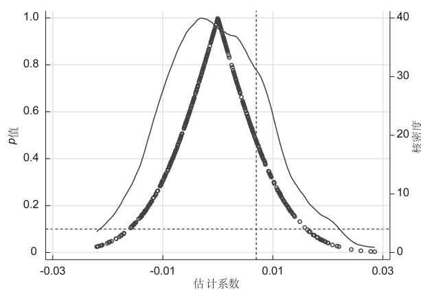
图2 安慰剂检验
