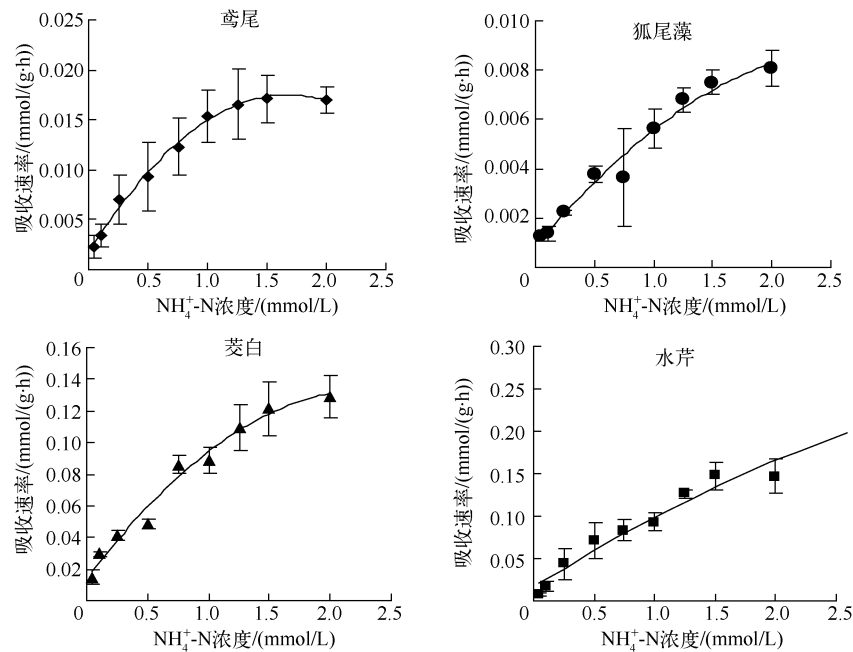
图 2 水生植物吸收 \text{NH}_4^+\text{-N} 动力学曲线
