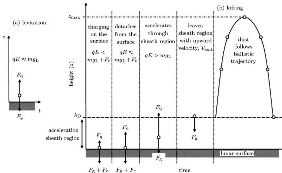
图 1 月尘静态悬浮模型和动态喷泉模型对比
