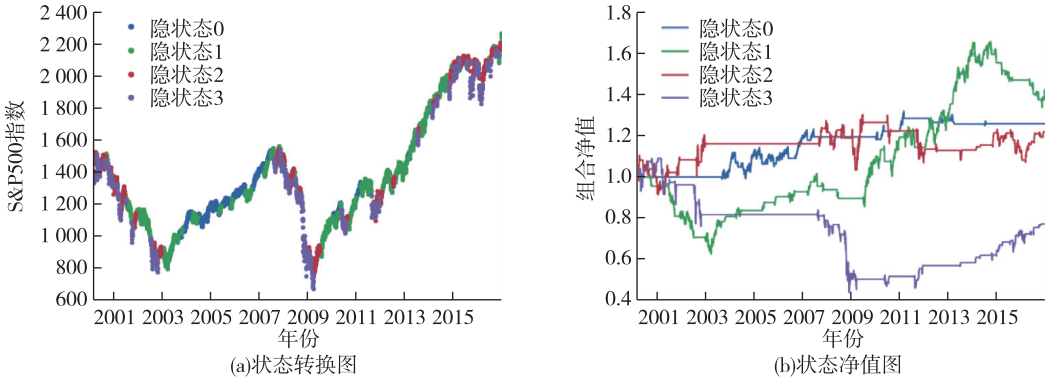
图 7 S&P 500 指数 4 状态 HMM 模型 Fig. 7 4-states HMM model for S&P 500 index
