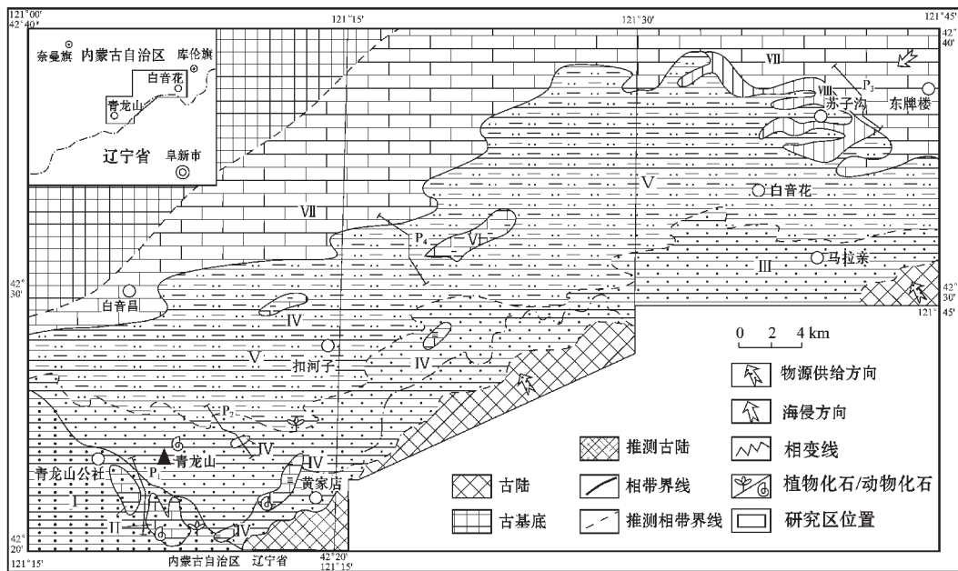
图1 内蒙古通辽南部石炭纪岩相古地理图
